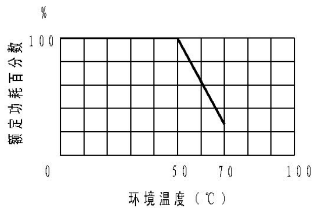
功率温度表
